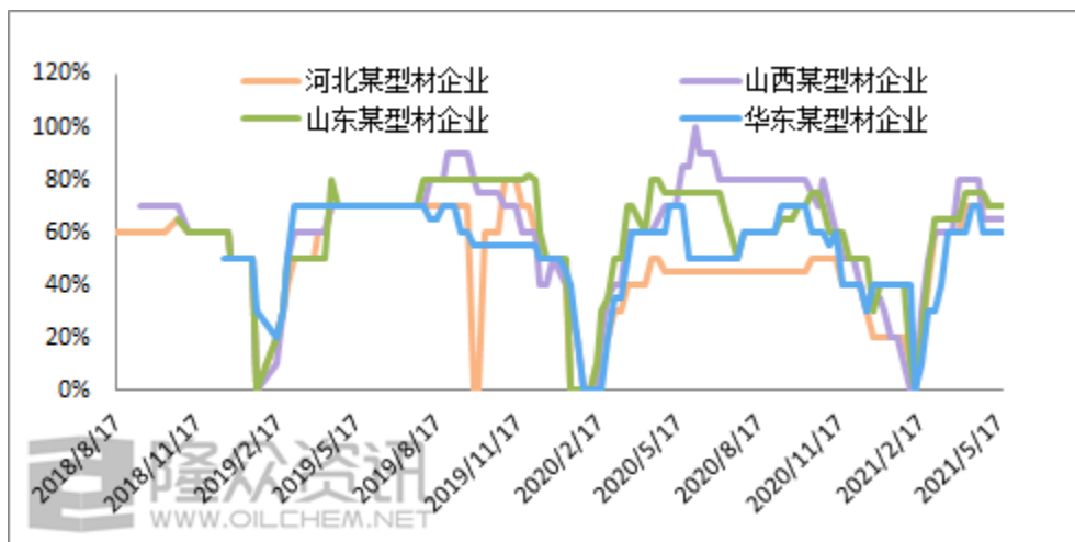
图 2018-2021 年 PVC 开工
